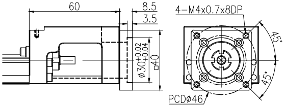
KKU50-F1(台达/三菱/安川/汇川/富士100W电机)
